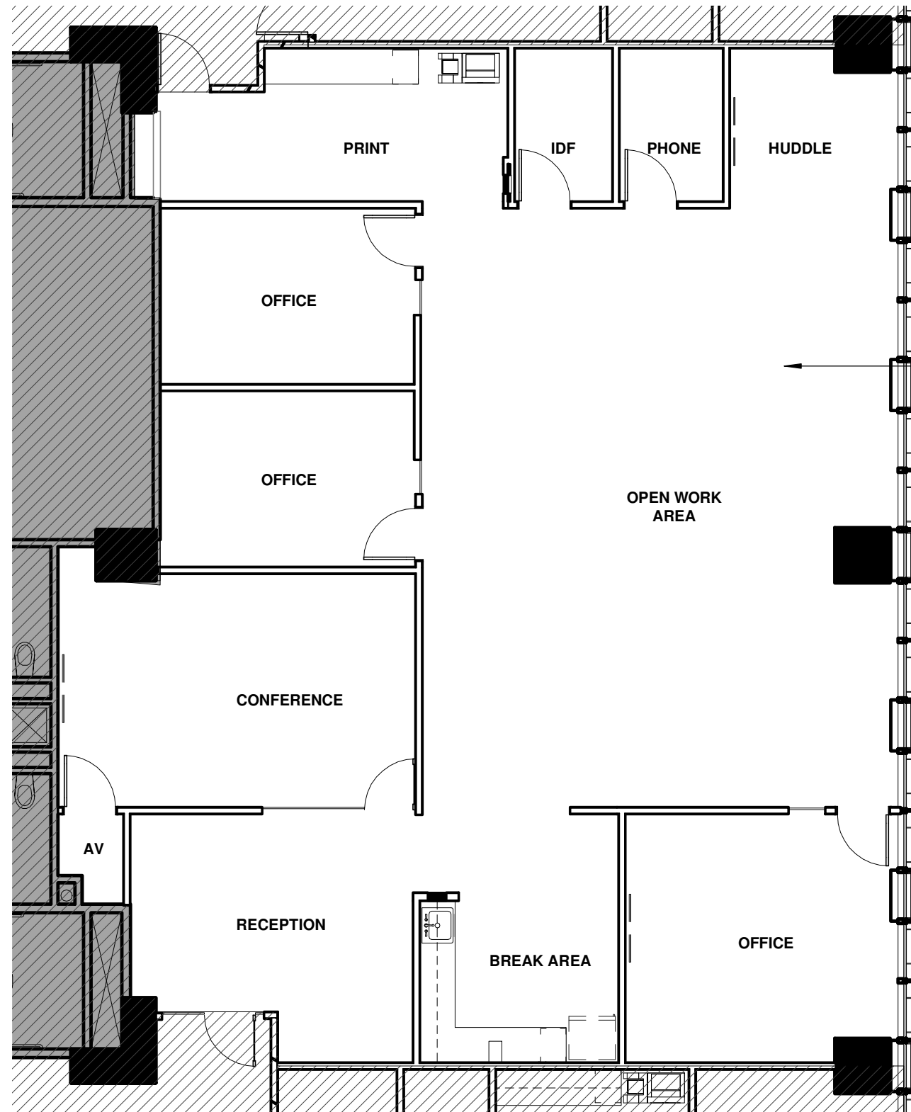
1 1/8" = 1'-0"
